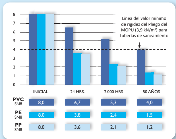
EVOLUCIÓN DE LA RIGIDEZ RCE = (E c )/D m 3 CON EL TIEMPO SEGÚN LA NORMA DIN 16961
