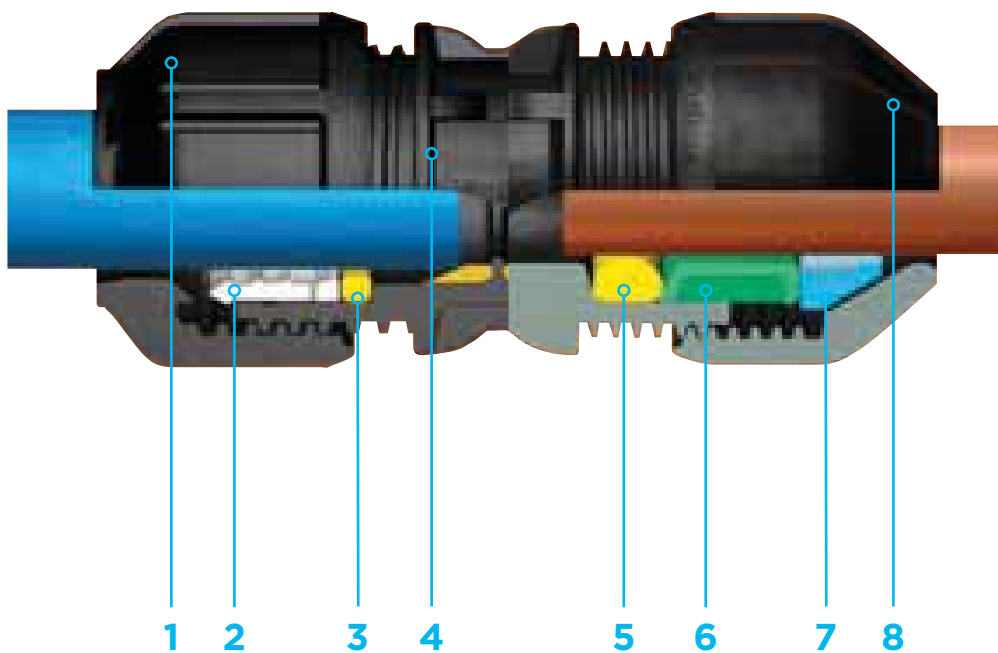
Conexión tubo PE
