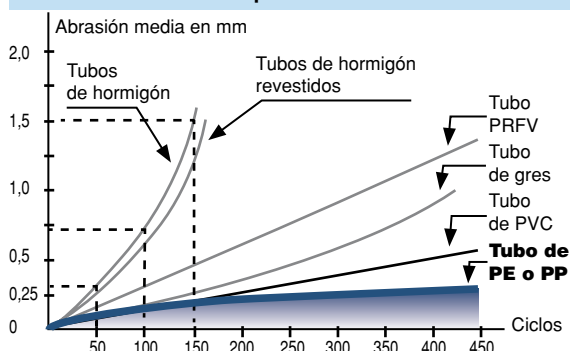
Curvas de abrasión para varios tipos de materiales de acuerdo con el procedimiento Darmstadt
